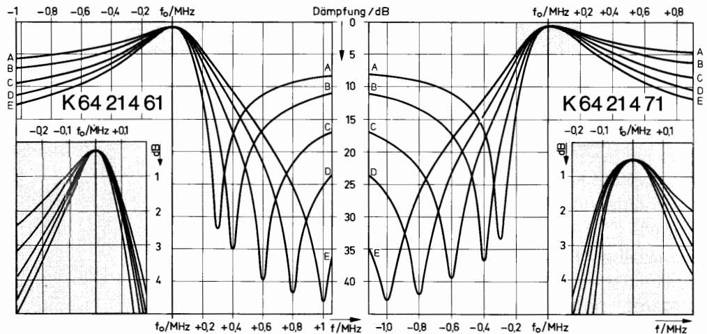
Durchlaßfrequenz unterhalb Sperrfrequenz
